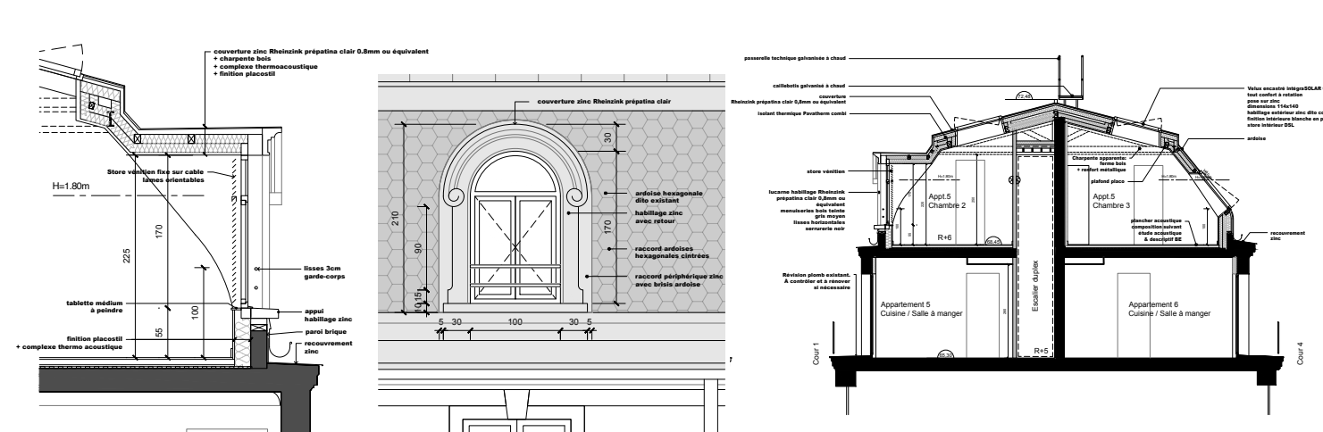
Détail lucarne projet - Coupe & élévation - 1/20e
