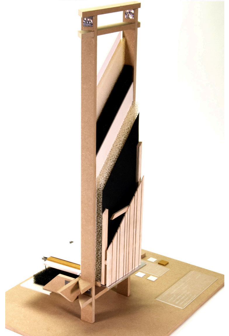
Maquette détail constructif Composition du Mur
