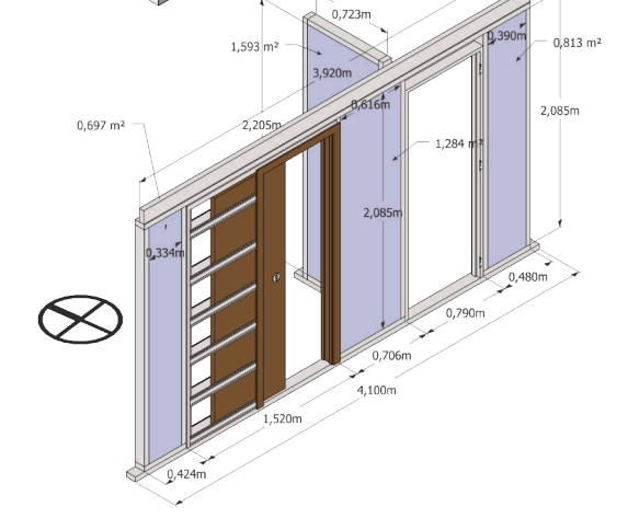
Réaménagement d'un atelier. Description détaillé des opérations - Axonométrie.
