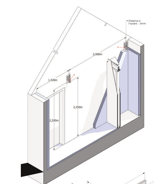
Maison individuelle neuve - ossature bois / isolation paille. Support de communication avec le charpentier.
