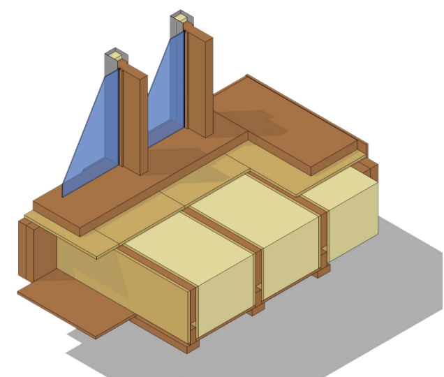
Réaménagement d'un atelier. Description détaillé des opérations - Axonométrie.
