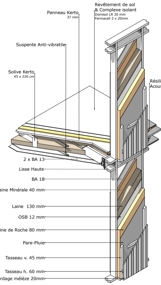
Analyse détails constructifs jonction mur-plancher Axonométrie Sketchup Coupe Autocad
