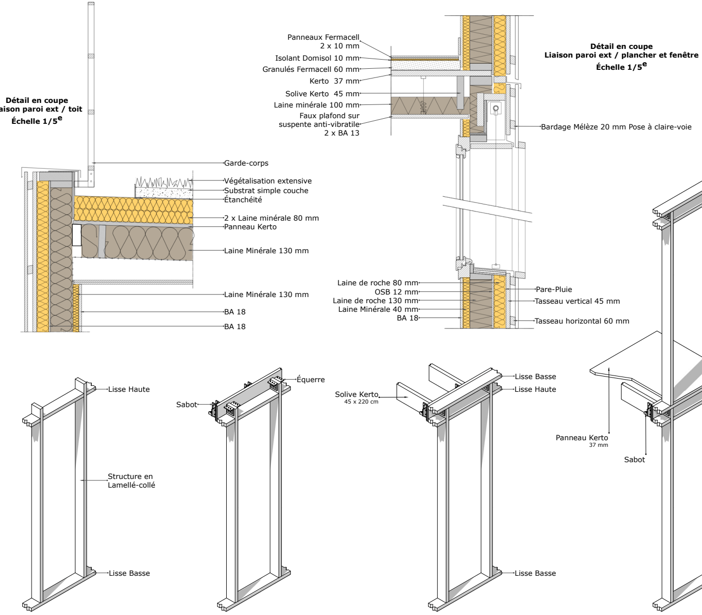
Analyse détails constructifs jonction mur-plancher Axonométrie Sketchup Coupe Autocad
