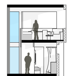
Coupe Transversale
