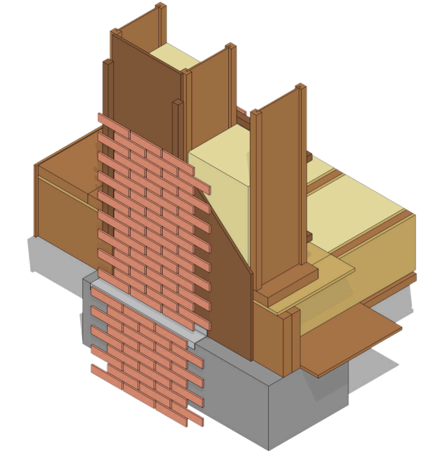
Maison individuelle neuve - ossature bois / isolation paille. Support de communication avec le charpentier.
