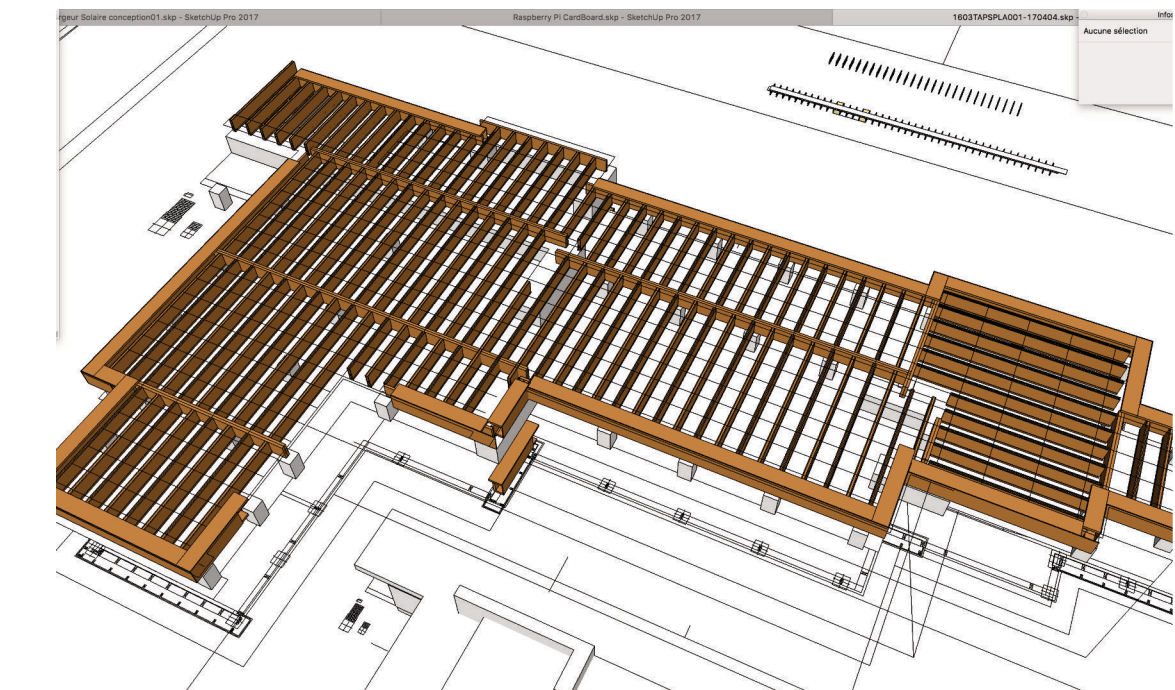
Maison individuelle neuve - ossature bois / isolation paille. Support de communication avec le charpentier.
