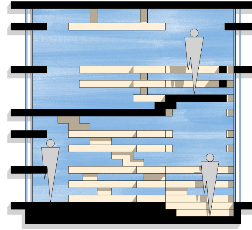
Coupe transversale depuis la façade
