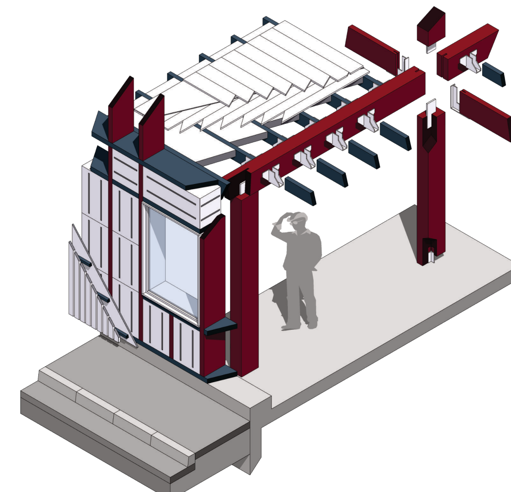
Axonométrie du principe constructif
